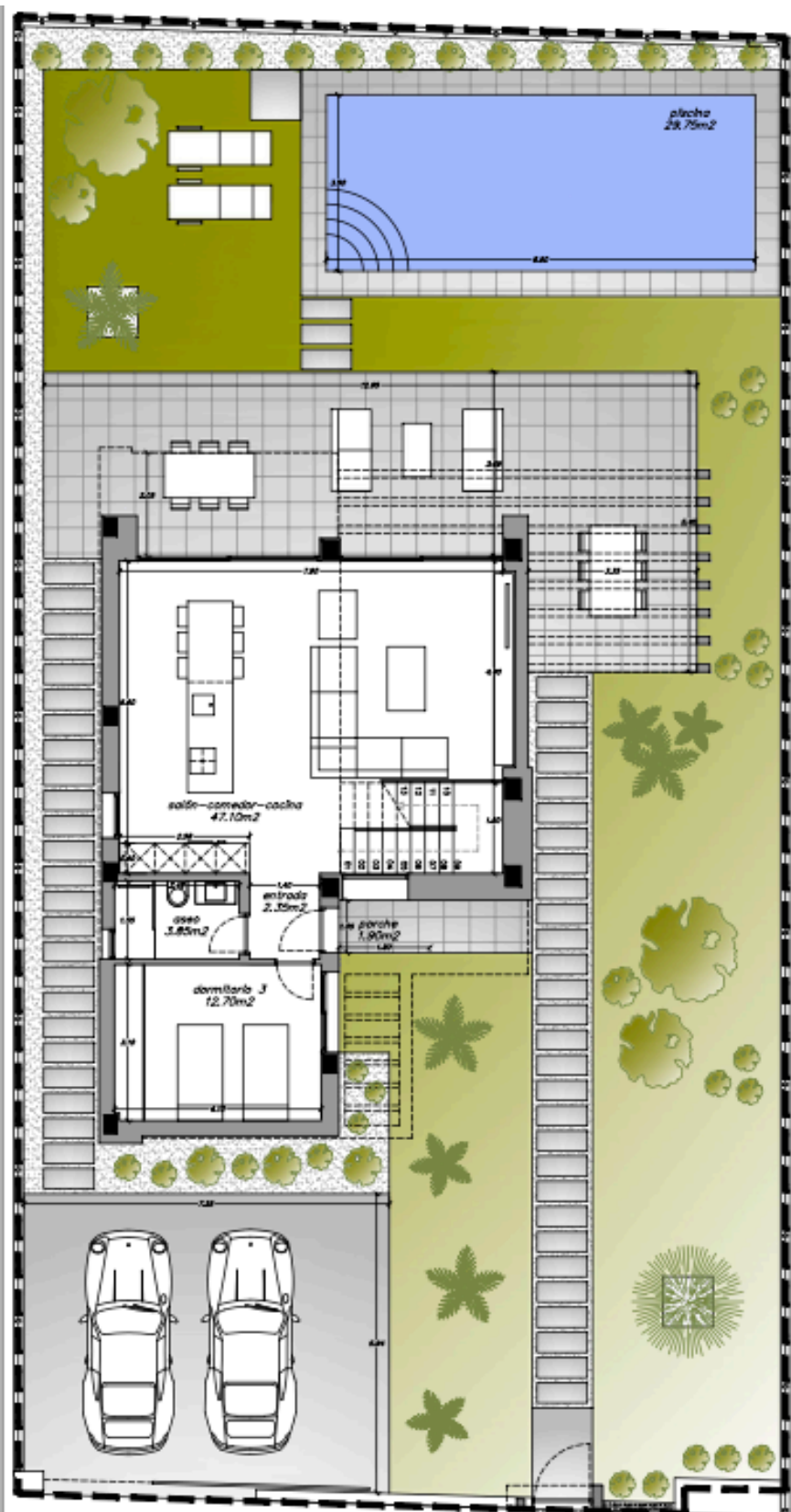
VIVIENDA 8 - CHALET UNIFAMILIAR TIPO 2 ESCALA GRÁFICA 1/100
