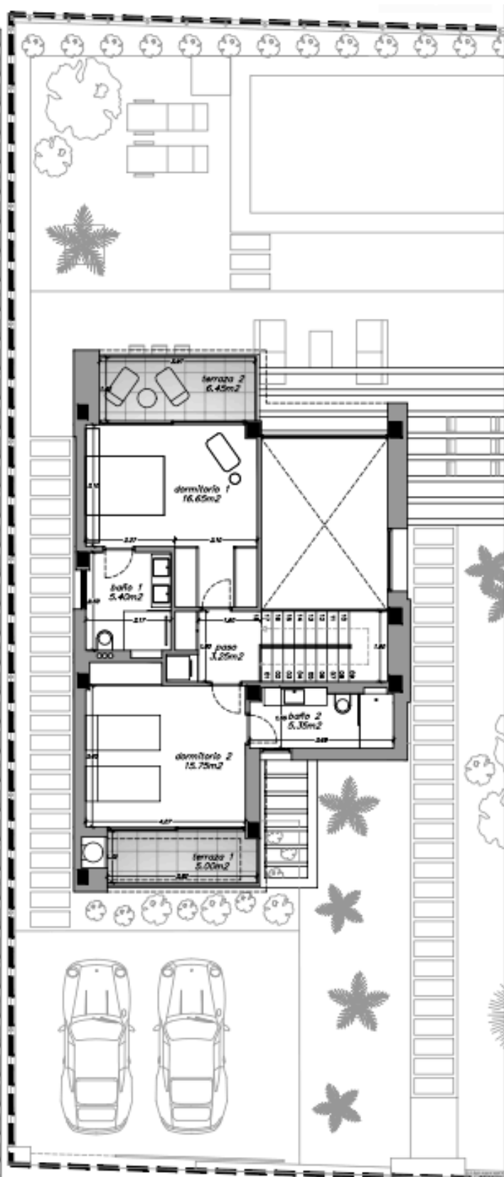
VIVIENDA 8 - CHALET UNIFAMILIAR TIPO 2 ESCALA GRÁFICA 1/100
