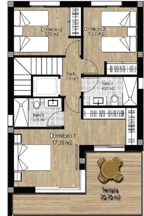
PLANTA PRIMERA
